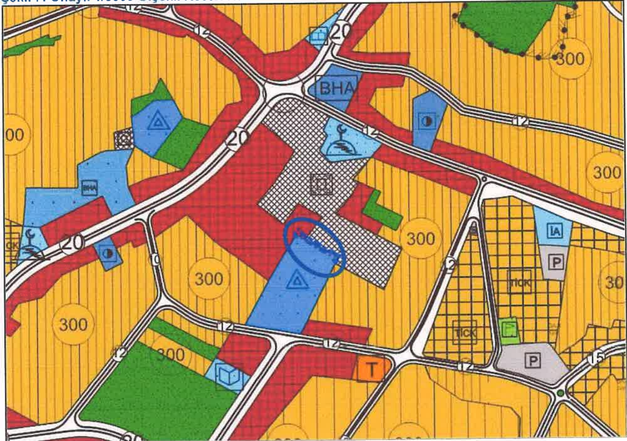
Şekil 7: Onaylı 1/5000 Ölçekli Kestel Nazım İmar Planı
